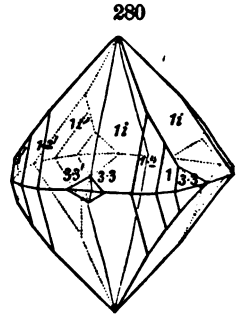
Scheelite.
